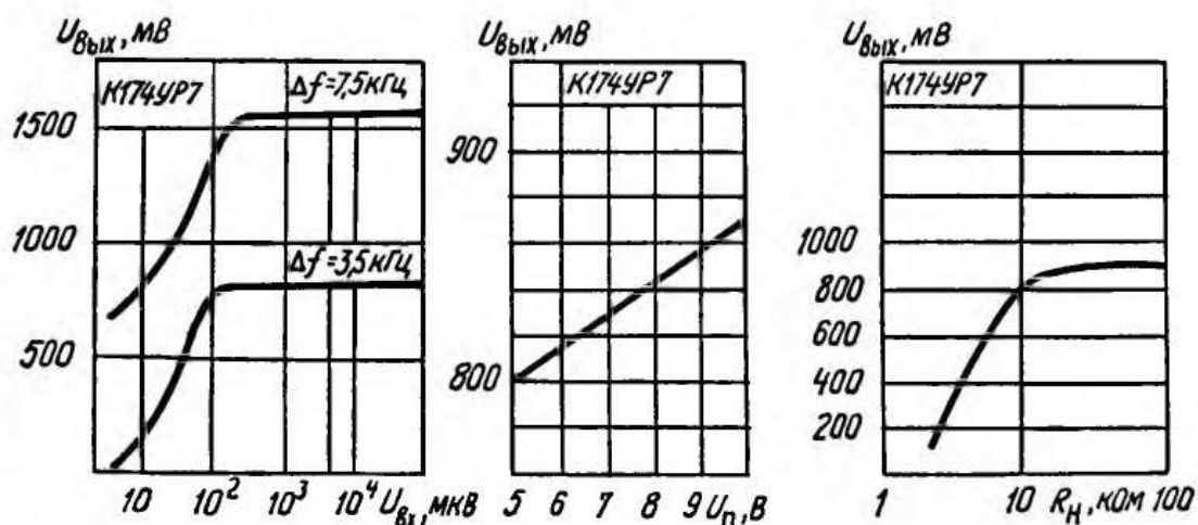
Основные характеристики ИМС К174УР7
