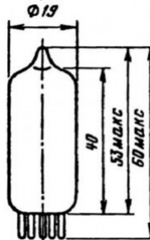
Чертёж лампы 6K4П:
