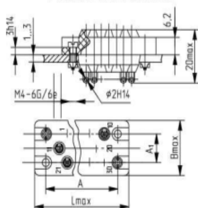
Рисунок 8 Розетка РП10 с замками
