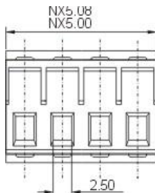
2EDGK-5.0 2EDGK-5.08
