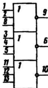
Условное графическое обозначение К564ЛЕ10
