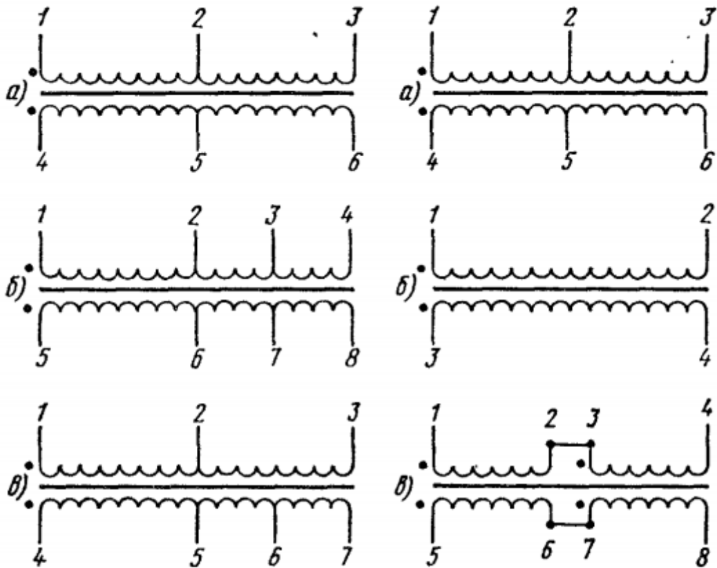
Рис. 9.4. Принципиальные электрические схемы низкочастотных согласующих трансформаторов: a — Т0Т1—Т0Т35; б — Т0Т36— Т0Т189; в — Т0Т202—Т0Т219
