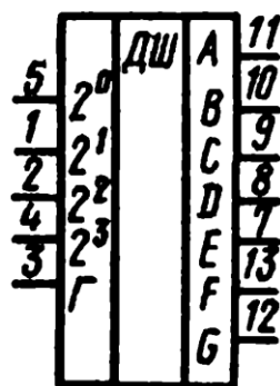
Условное графическое обозначение К514ИД2, КР514ИД2
