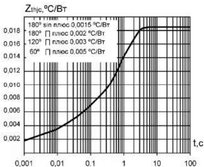
Рис. 2. Переходное тепловое сопротивление переход-корпус ( постоянный ток )
