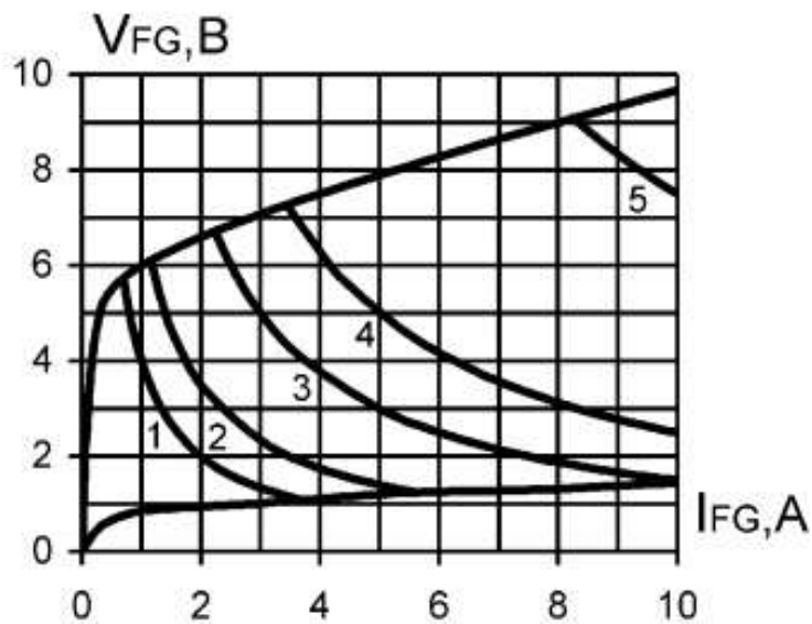
Рис. 3. Предельные характеристики цепи управления
