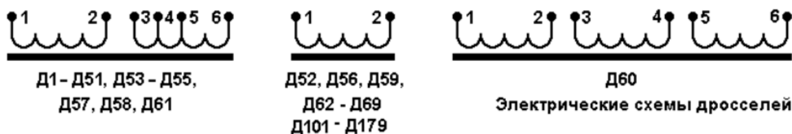
Схема обмоток дросселей Д1-Д69, Д101-Д179
