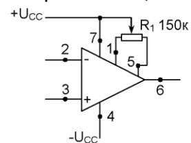
Схема внешней балансировки напряжения смещения
