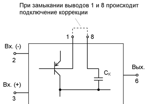
Организация внутренней частотной коррекции К/КР544УД2
