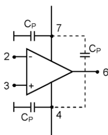
Вариант развязки К/КР544УД2 по цепям питания
