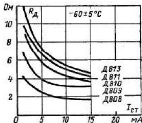
Зависимости дифференциального сопротивления от тока
