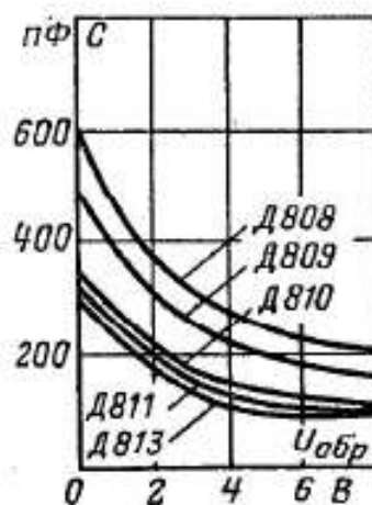
Зависимости емкости от напряжения
