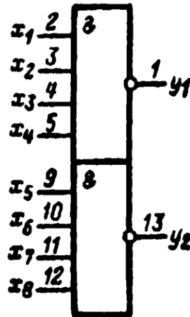
Условное графическое обозначение К176ЛА8
