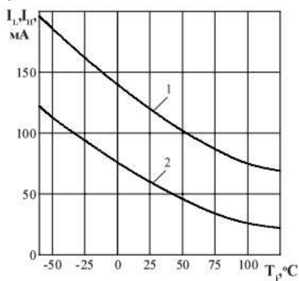
Рисунок 11 - Зависимость тока удержания I_H (1) и тока включения I_T (2) от температуры перехода T_j .
