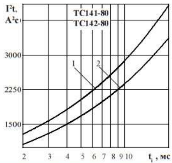
Рисунок 6 - Зависимость защитного показателя \Gamma t от длительности импульса тока t_1 при исходной температуре структуры T_j = 25\text{ }^\circ\text{C} (1) и максимальной температуре T_{jm} (2)
