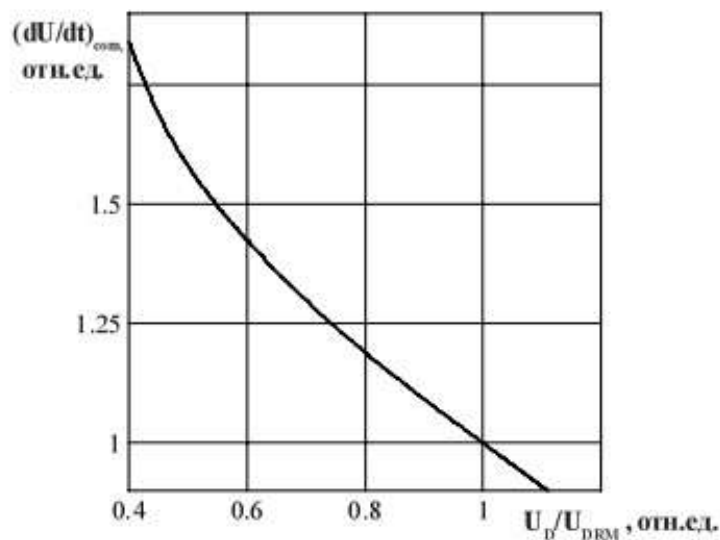
Рисунок 13 - Зависимость критической скорости нарастания коммутационного напряжения (dU_D/dt)_{crit} (отн.ед.) от величины приложенного напряжения U_D/U_{DRM} (отн.ед.) при I_T = I_{TRMS} , T_j = 125^\circ\text{C} , t_l = 10 мс.
