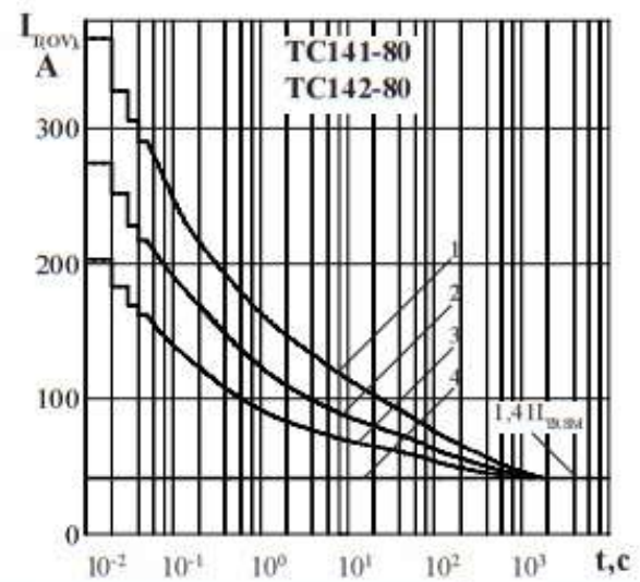
Рисунок 7 - Зависимость допустимой амплитуды тока перегрузки в открытом состоянии I_{rov} синусоидальной формы частотой f = 50\text{ Гц} от длительности перегрузки t при естественном охлаждении на типовом охладителе при отношении тока, предшествующего перегрузке, I_T к максимально допустимому действующему току триака I_{TRMS} равному k = I_T / I_{TRMS} : k = 0 (1); 0,5 (2); 0,75 (3); 1,0 (4).
