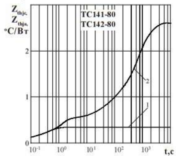
Рисунок 8 - Зависимость переходного теплового сопротивления переход - корпус Z_{thjc} (1) и переход-среда Z_{thja} (2) от времени t при естественном охлаждении на типовом охладителе при температуре окружающей среды T_a = 40\text{ }^\circ\text{C} .
