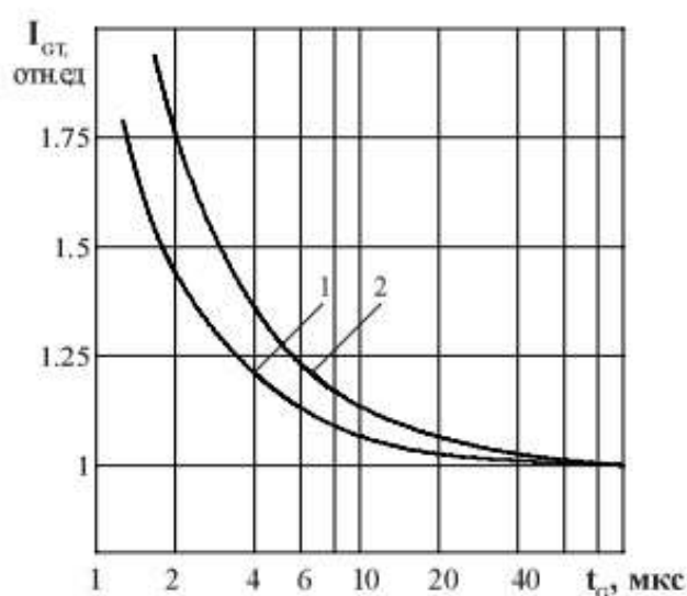
Рисунок 10 - Зависимость отпирающего импульсного тока управления I_{OT} от длительности управляющего импульса t_G при температуре перехода T_j = 25^\circ\text{C} (1), T_{jmin} = \text{минус } 50^\circ\text{C} (2) и напряжения в закрытом состоянии U_D = 12\text{ В} .
