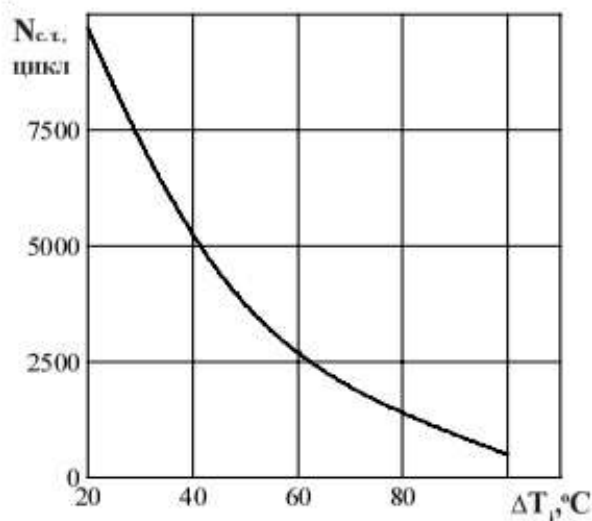
Рисунок 15 - Зависимость допустимого числа циклов N_{c.t.} от перепада температуры структуры \Delta T_j при циклической токовой нагрузке.
