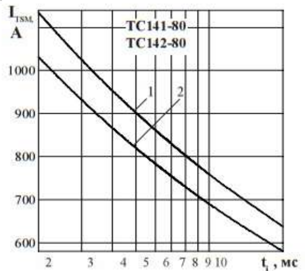
Рисунок 5 - Зависимость допустимой амплитуды ударного тока в открытом состоянии I_{TSM} от длительности импульса тока t_i при исходной температуре структуры T_i = 25 °C (1) и максимальной температуре T_m (2)
