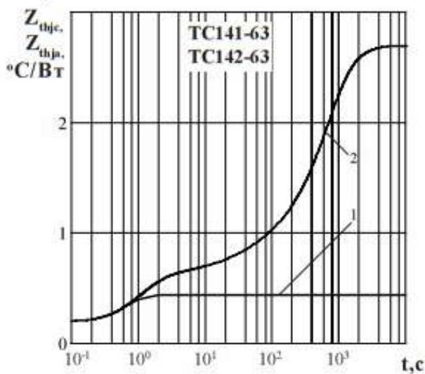
Рисунок 8 - Зависимость переходного теплового сопротивления переход - корпус Z_{thjc} (1) и переход-среда Z_{thja} (2) от времени t при естественном охлаждении на типовом охладителе при температуре окружающей среды T_a = 40\text{ }^\circ\text{C} .
