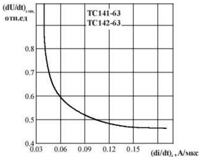
Рисунок 14 - Зависимость критической величины скорости нарастания коммутационного напряжения (dU/dt)_{crit} от скорости спада предшествующего тока в открытом состоянии (di_i/dt)_i при амплитуде предшествующего тока в открытом состоянии I_T = I_{TRSM} и максимально допустимой температуре перехода T_{jм} .
