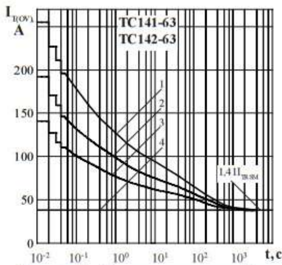
Рисунок 7 - Зависимость допустимой амплитуды тока перегрузки в открытом состоянии I_{rov} синусоидальной формы частотой f = 50\text{ Гц} от длительности перегрузки t при естественном охлаждении на типовом охладителе при отношении тока, предшествующего перегрузке, I_T к максимально допустимому действующему току триака I_{TRMS} равному k = I_T / I_{TRMS} : k = 0 (1); 0,5 (2); 0,75 (3); 1,0 (4).
