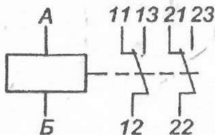
Электрическая принципальная схема
