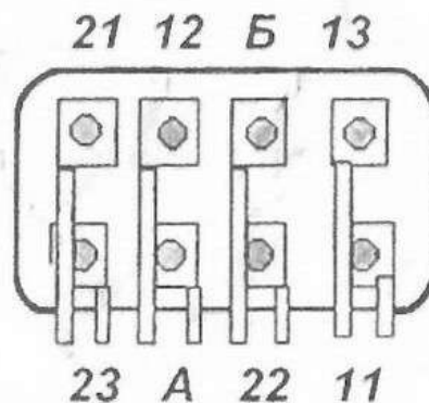
Расположение выводов контактов и обмоток
