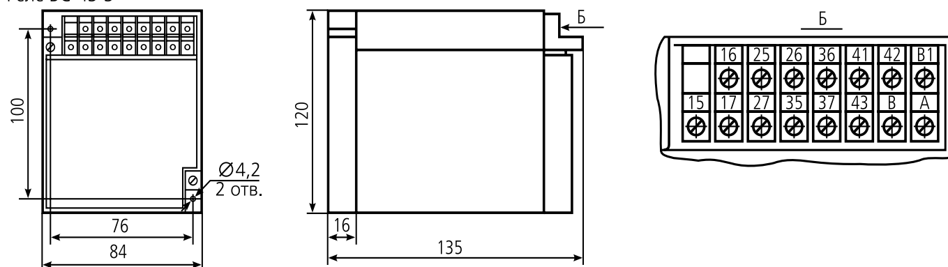
Реле BC-43-3
