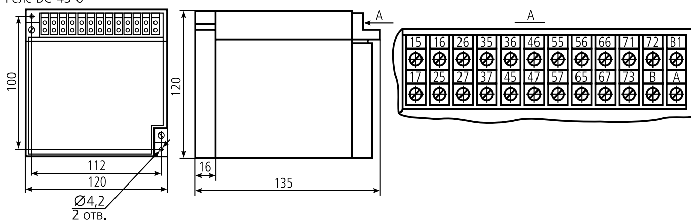
Реле BC-43-6
