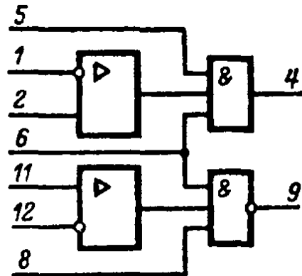
Условное графическое обозначение К170УП1
