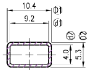
A-A Section
