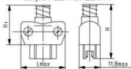
Рисунок 4 Вилка в угловом металлическом кожухе или в угловом пластмассовом кожухе РШ2Н-1, РШ2НП-1
