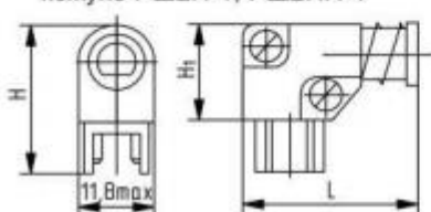
Рисунок 4 Вилка в угловом металлическом кожухе или в угловом пластмассовом кожухе РШ2Н-1, РШ2НП-1
