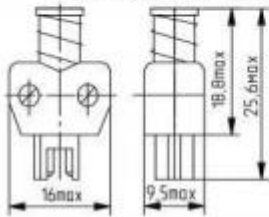
4-контактная вилка в литом металлическом или пластмассовом прямом кожухе РШ2Н-5, РШ2НП-5
