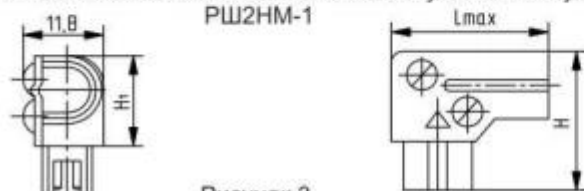
Рисунок 3 Вилка в прямом металлическом кожухе или в прямом пластмассовом кожухе РШ2Н-1, РШ2НП-1
