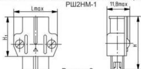
Рисунок 2 Вилка в штампованно-литом металлическом угловом кожухе РШ2НМ-1
