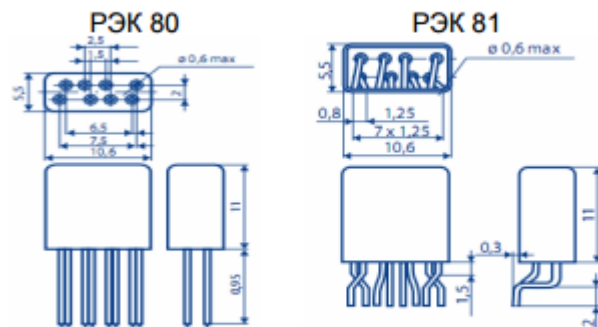
Габаритные размеры
