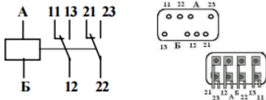
Схема электрическая принципиальная РЭК 80, РЭК 81
