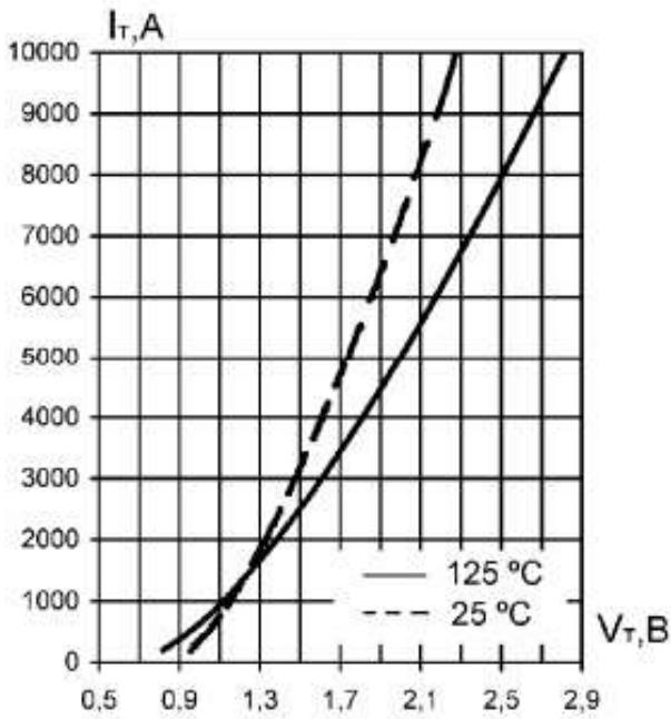
Рис. 1. Предельные вольт-амперные характеристики в открытом состоянии
