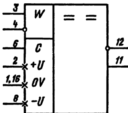
Условное графическое обозначение K597CA1, KM597CA1, KP597CA1, KC597CA1
