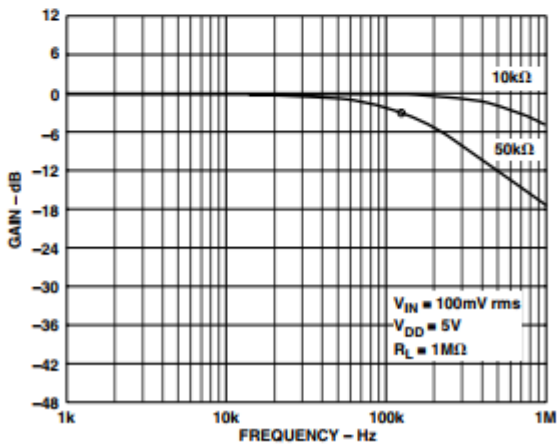
TPC 20. AD5200 -3 dB Bandwidth
