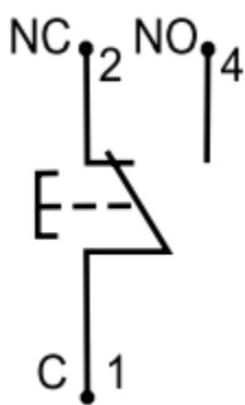
Схема подключения
