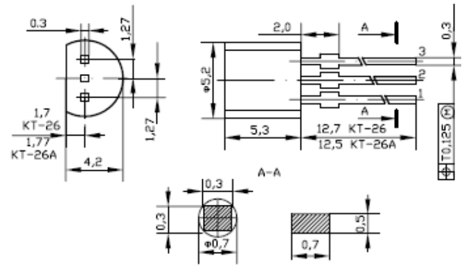
Корпус КТ-26
